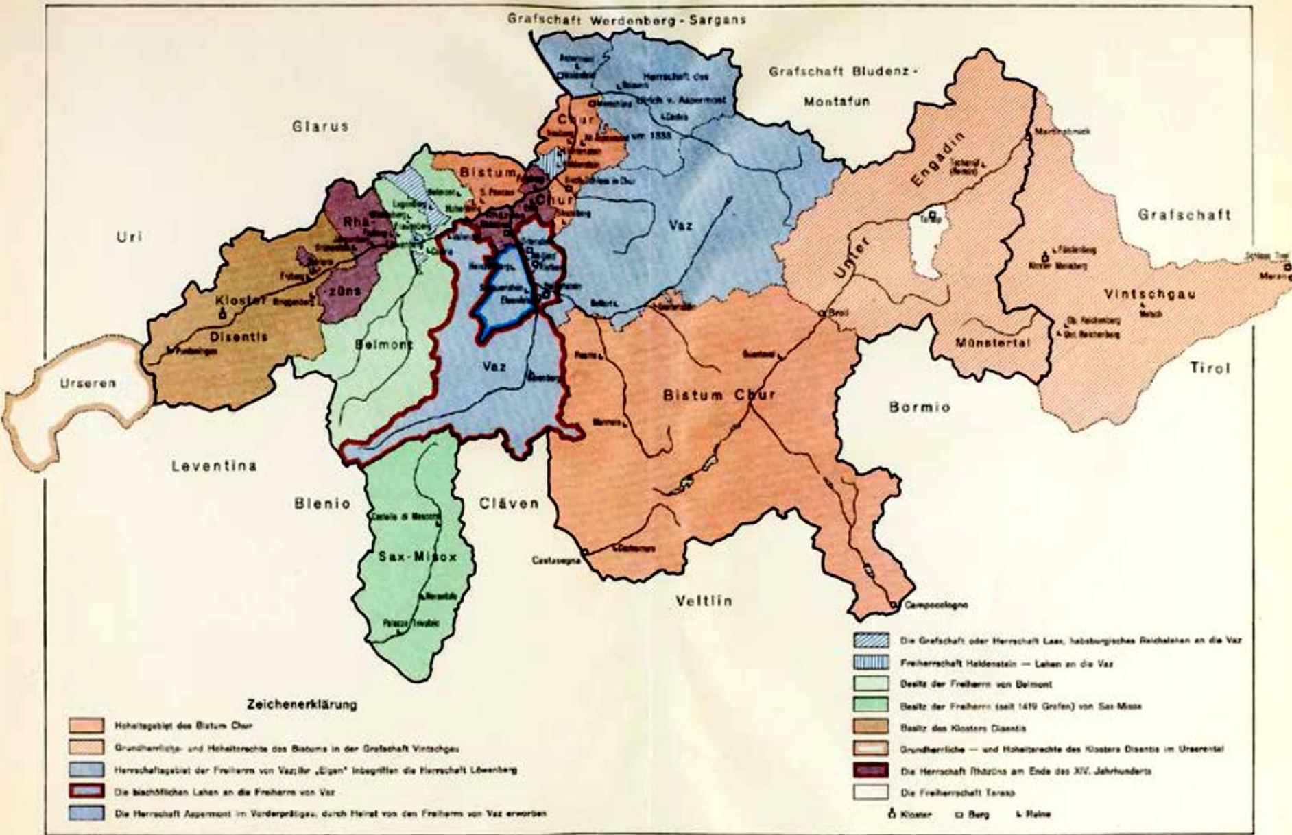
GRAUBÜNDEN IN DER FEUDALZEIT Die Territorialherrschaften um 1337 beim Tode des Freiherren Donat von Vaz
